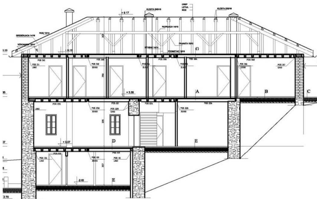
Фазе реконструкције централног конака у манастиру Девич (почетно стање, консолидација, радови на обнови – зима 2007) Скице доле: пресек новог конака и пресек основе другог спрата
