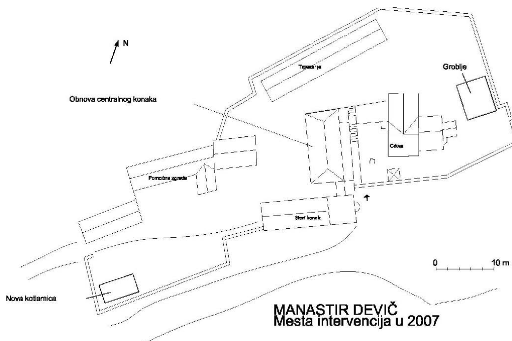
Реконструисани централни конак у манастиру Девич
