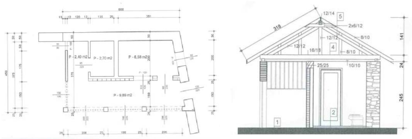
Помоћна зграда – хоризонтални и попречни пресек
