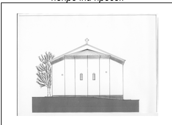
источна фасада
