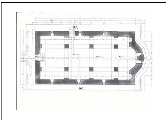
основа цркве
