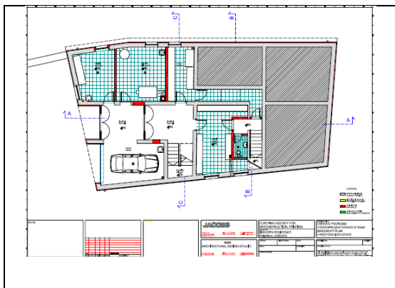
основа подрума
