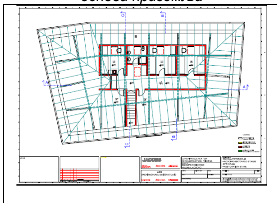
основа поткровља
